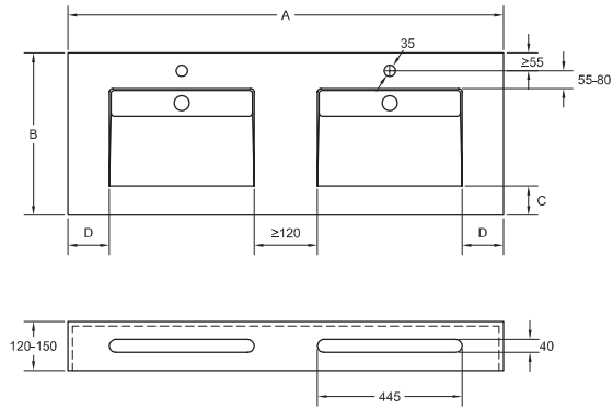
*Dimensions pour siphon Quare
