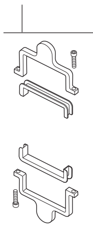
RP63688 Mounting Plates, Sleeves & Screws Chapas de instalación, Casquillos y Tornillos Plaques de montage, manchons et vis
