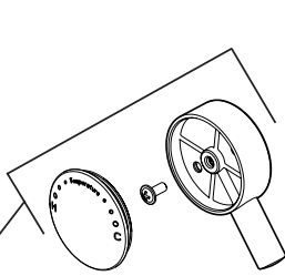
RP49096▲ Temperature Knob, Cover & Screw Perilla de la Temperatura, Cubierta y Tornillo Poignée de réglage de température et vis
